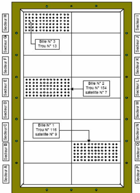
Exemple de repérage
