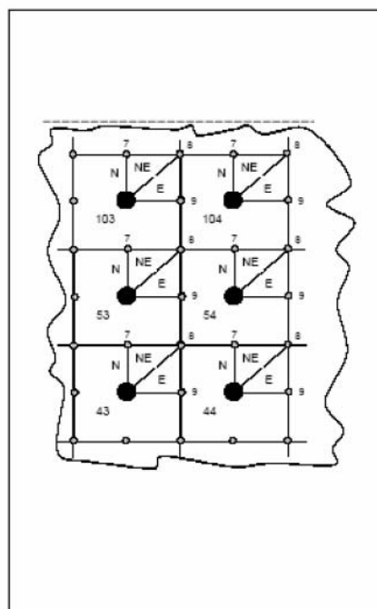
Disposition des satellites sur gabarit de repérage
